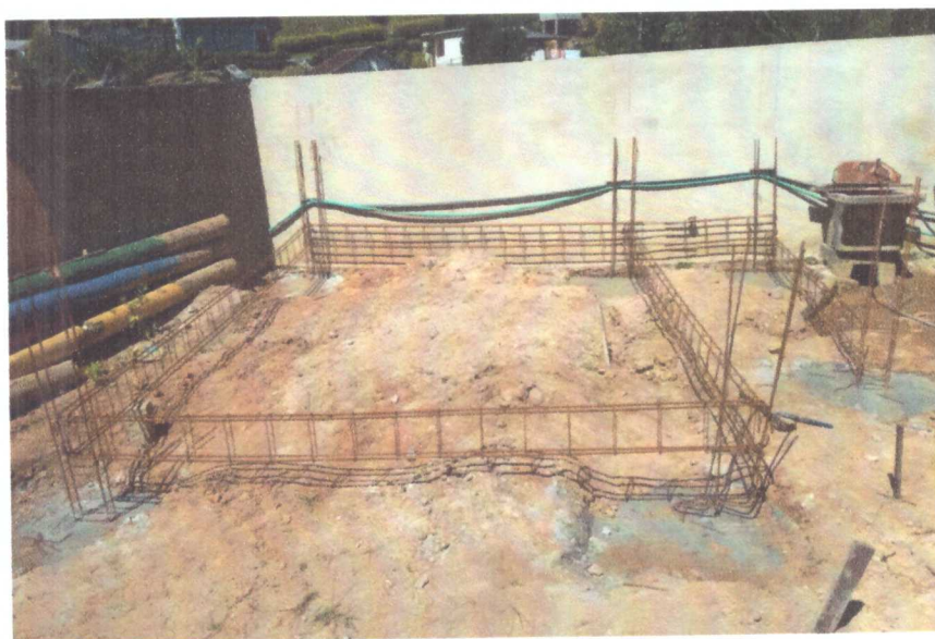
ARMAÇÃO DE AÇO DA FUNDAÇÃO DA SALA DO MATERNAL E BANHEIRO
